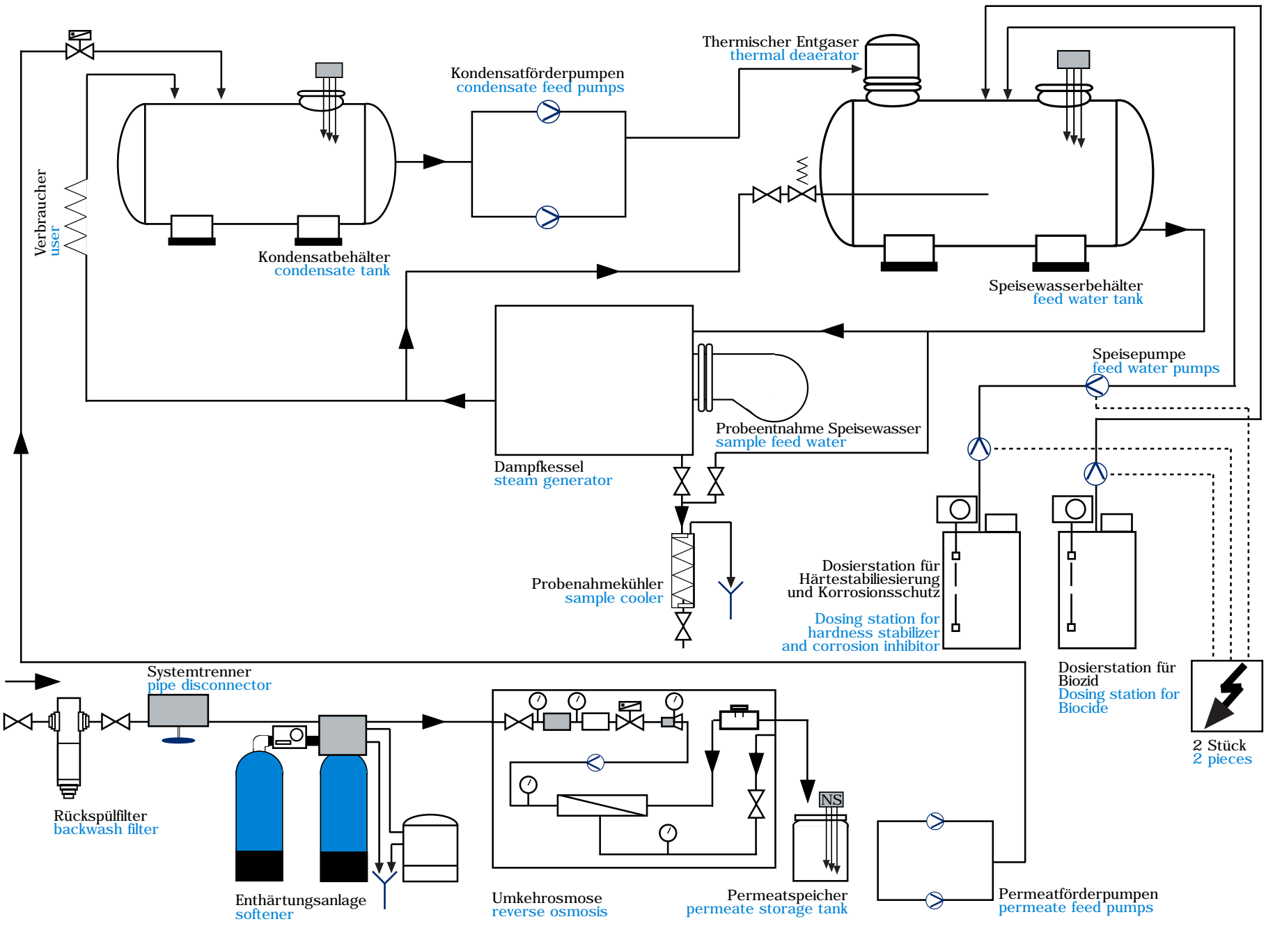
CWG - Verfahrensschema - Kesselwasseraufbereitung CWG - Process diagram - Boiler feed water treatment
